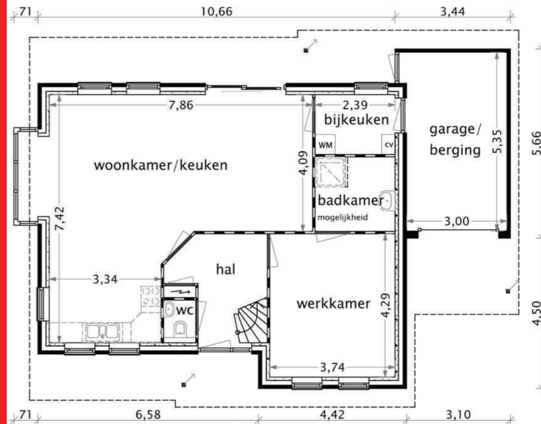
Beganegrond
